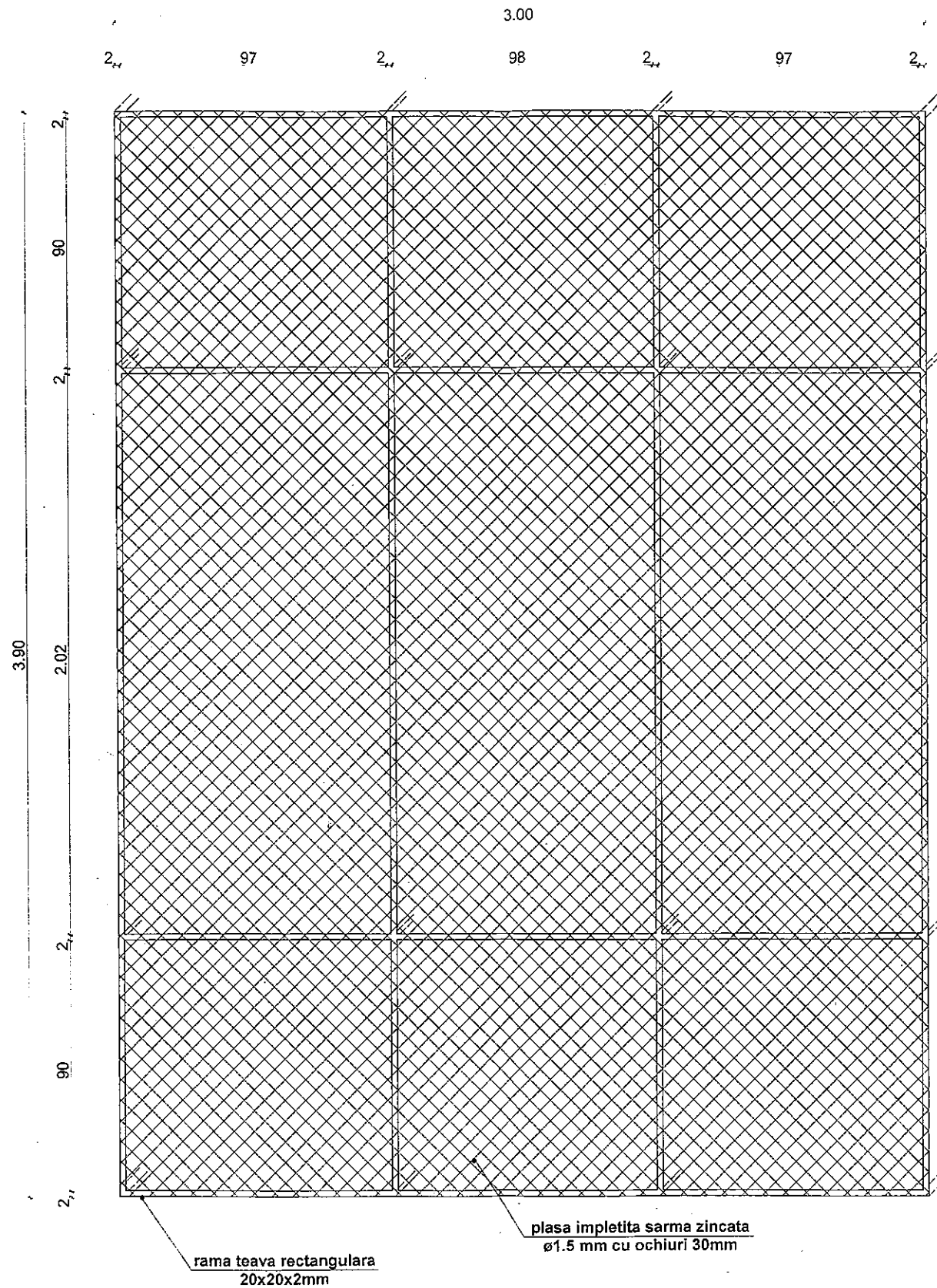
VEDERE SCARA 1:20
